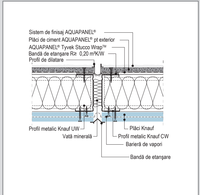
W384E-BFU2.ro Rost de dilatație structural
