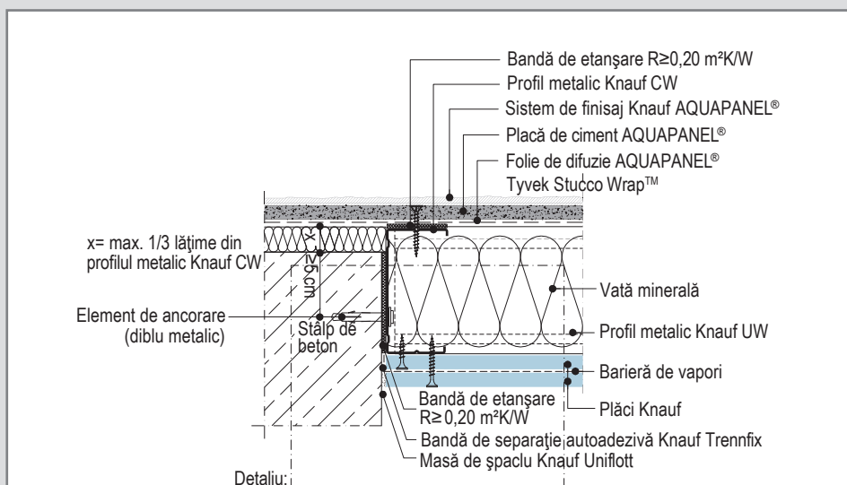
W384E-B1.ro Secțiune transversală cu îmbinarea plăcilor
