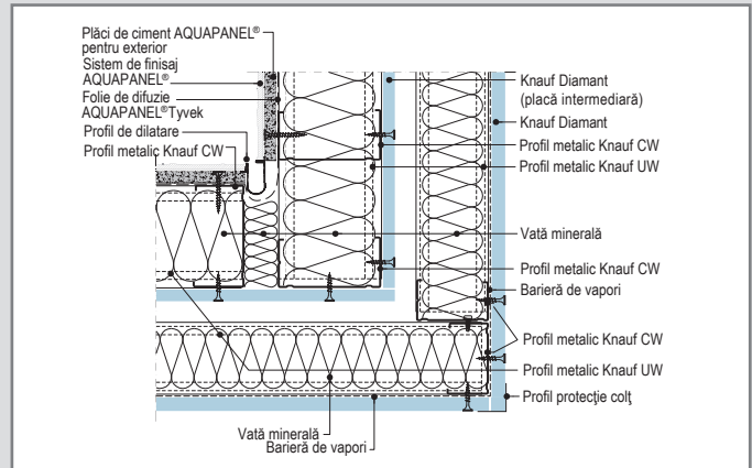
W378E-DBFU1.ro Realizare colț interior cu profil de dilatare
