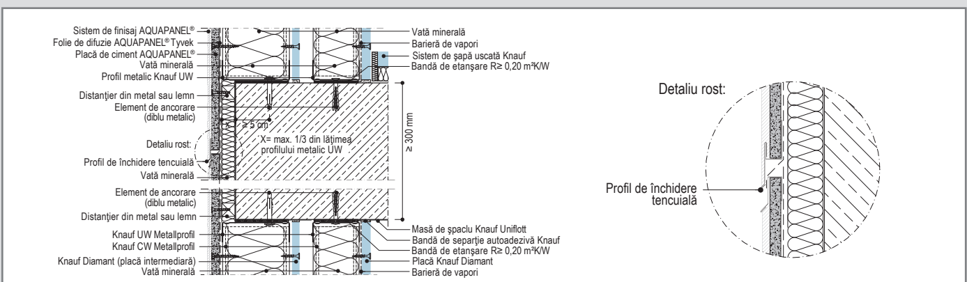
W378E-VM1.ro Realizare rost de dilatare orizontal
