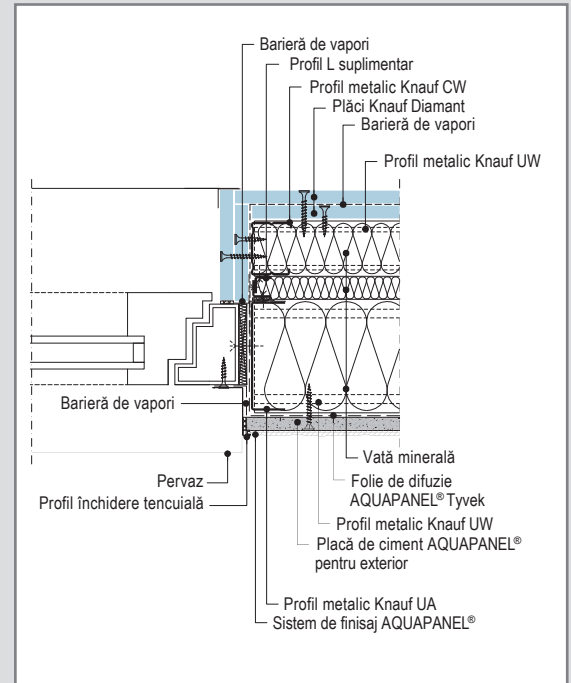
W388E-FE-VM2.ro Detaliu racord la fereastră - secțiune orizontală, varianta 2
