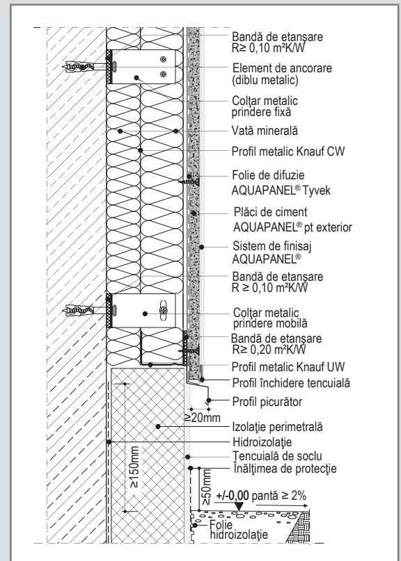
W684T-SO-V2.ro Fațadă cortină - detaliu soclu
