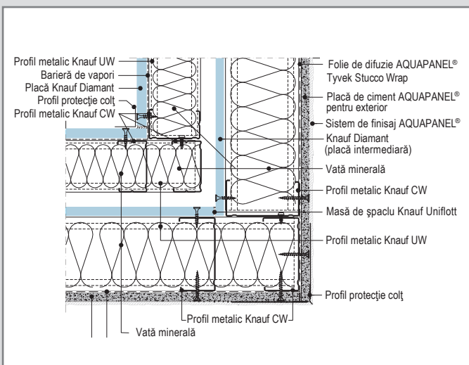
W378E-E1.ro Realizare colț exterior
