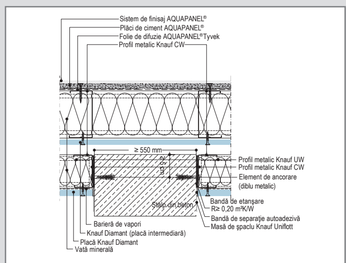
W378E-HS1.de Trecere și racord la stâlpul din beton
