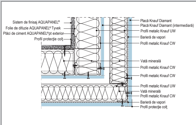
W378E-D1.ro Realizare colț interior
